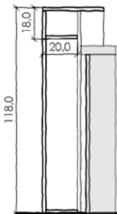
Thekenquerschnitt Seattle
