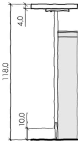
Thekenquerschnitt London
