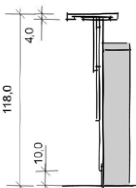
Thekenquerschnitt Santorin
