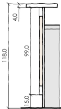
Thekenquerschnitt Belfast
