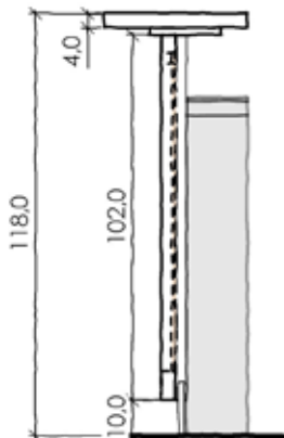
Thekenquerschnitt Rosenheim
