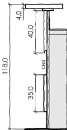
Thekenquerschnitt Riga
